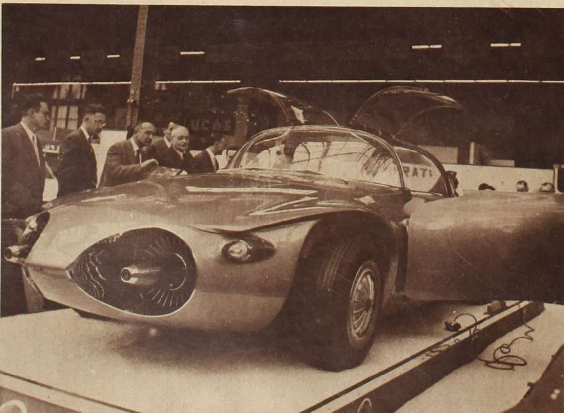
Die Geschichte des Automobils in siebzig Jahren demonstrieren diese beiden Wagen: der im Pariser Autosalon ausstellte amerikanische Turbinenwagen „Feuervogel II“ (oben) und das Benz-Modell aus dem Jahre 1885, das eben mit neun Stundenkilometern in die Kurve braust. Es mußte anlässlich der UNESCO-Museumswoche die wohlverdiente Pensionistenruhe für kurze Zeit unterbrechen.
