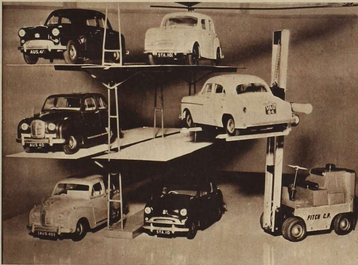
NACH DIESEM NEUEN GARAGENSYSTEM können bei einer gegebenen Grundfläche zwei- bis dreimal so viele Wagen untergebracht werden. Sie werden mit Hilfe eines Gabelstaplers auf Eisenbeton-Plattformen gehoben. Die Baukosten sollen sich pro Wagen auf S 9600 belaufen. Das Modell wurde auf der Industrieausstellung in Earls Court, London, gezeigt.
