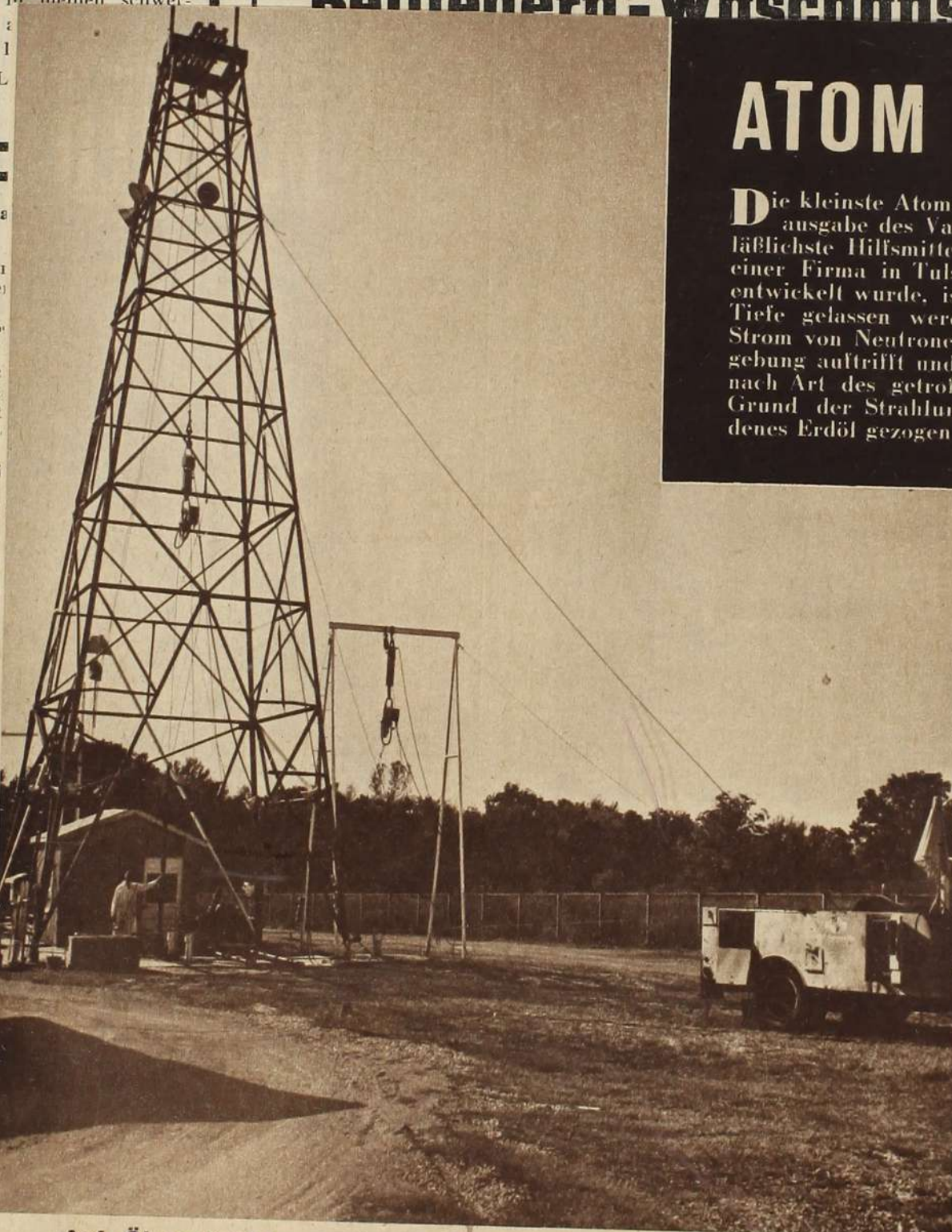
Auf Öl gestoßen war eine Bohrfirma bei Aufschlußbohrungen in einem Hoffungsgebiet im Südwesten der USA. Um den Umfang der neuen Ölvorkommen zu bestimmen, ließ man den Atomreaktor an die Bohrstelle bringen.
