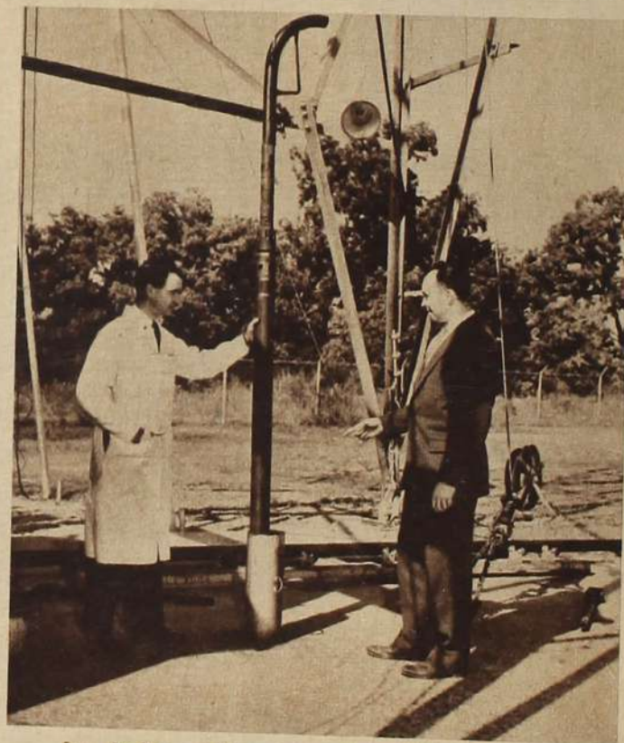
In jedes Standardbohrloch paßt der neue, röhrenförmige Miniaturreaktor, der trotz seinen kleinen Abmessungen die beachtliche Kapazität von 200.000 Volt hat.
