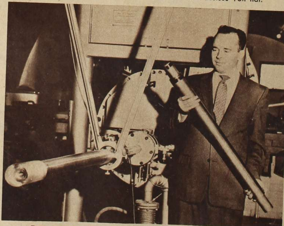
Der neue „Baby“-Reaktor kann von einem Mann leicht getragen werden. Das Gerät links daneben ist ein „ausgewachsener“ Van De Graaff-Reaktor, wie ihn heute bereits zahlreiche Firmen für Forschungszwecke verwenden.
