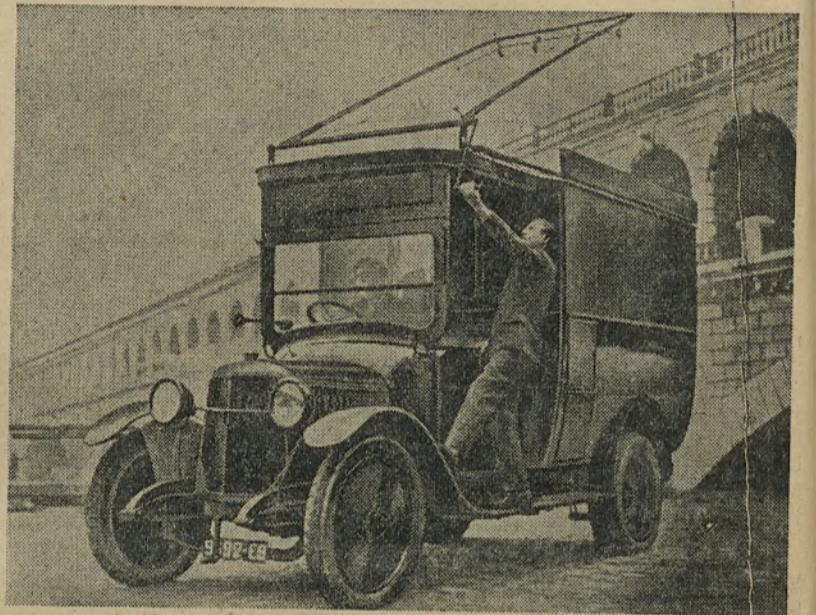
Radio im Dienste der Pariser Polizei. Das Bild zeigt einen mit Radio ausgestatteten Pariser Polizeiwagen. Auf dem Dach des Wagens befindet sich die aufklappbare Antenne.
