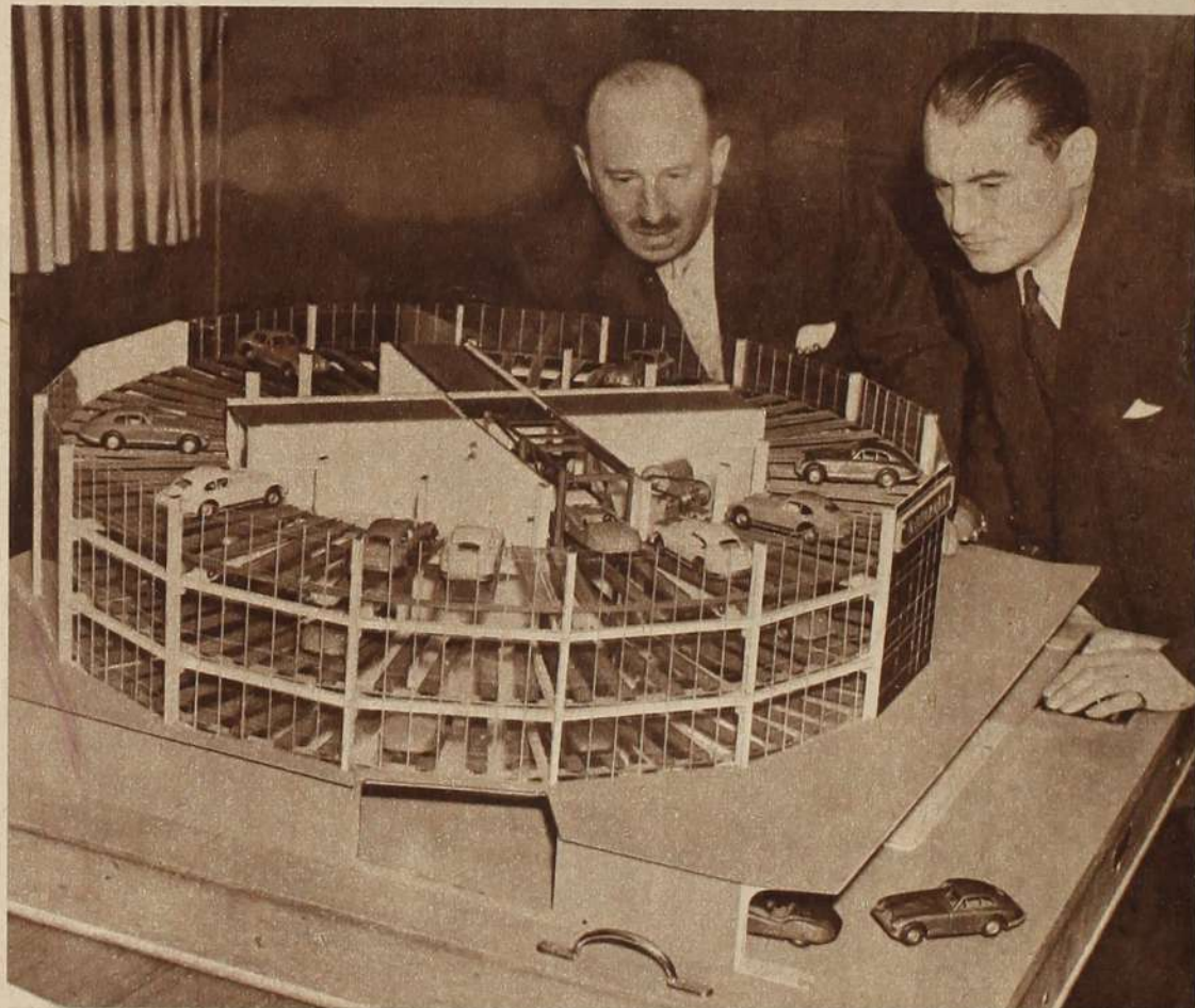
Englands erste rotierende Garage wird wahrscheinlich in der Nähe der South- wark-Brücke gebaut werden. Das von amerikanischen Technikern erdachte „Rotapark“- System funktioniert folgendermaßen: der Wagen wird in einen Lift und in das gewünschte Stockwerk gefahren, dann dreht sich die Garage, bis der Wagen in eine leere Box ausfahren kann. Die „Rückfahrt“ wird von einem Elektronengehirn automatisch gesteuert.
