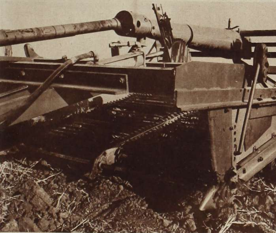
der ohne Scharen, sondern mit einer an deren Stelle verwendeten Gestänge-ten sich bestens bewährt. Die Grabstangen zerkleinern große Schollen und heben auf das Förderband, das meistens mit einem Gummibelag versehen ist.
