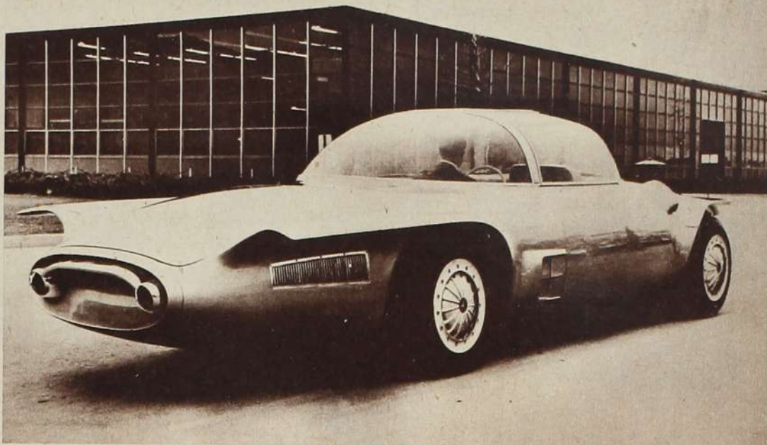
Das „Auto der Zukunft“ der General Motors Corp. ist mit einem Zweizylinder-250 PS-Freikolbenmotor ausgestattet. Die dem Zylinder dieses Doppelkolbenmotors entströmenden verbrannten Gase haben eine Temperatur von nur zirka 480 Grad Celsius. (Bei der Gasturbine: 800 bis 900 Grad Celsius.)
