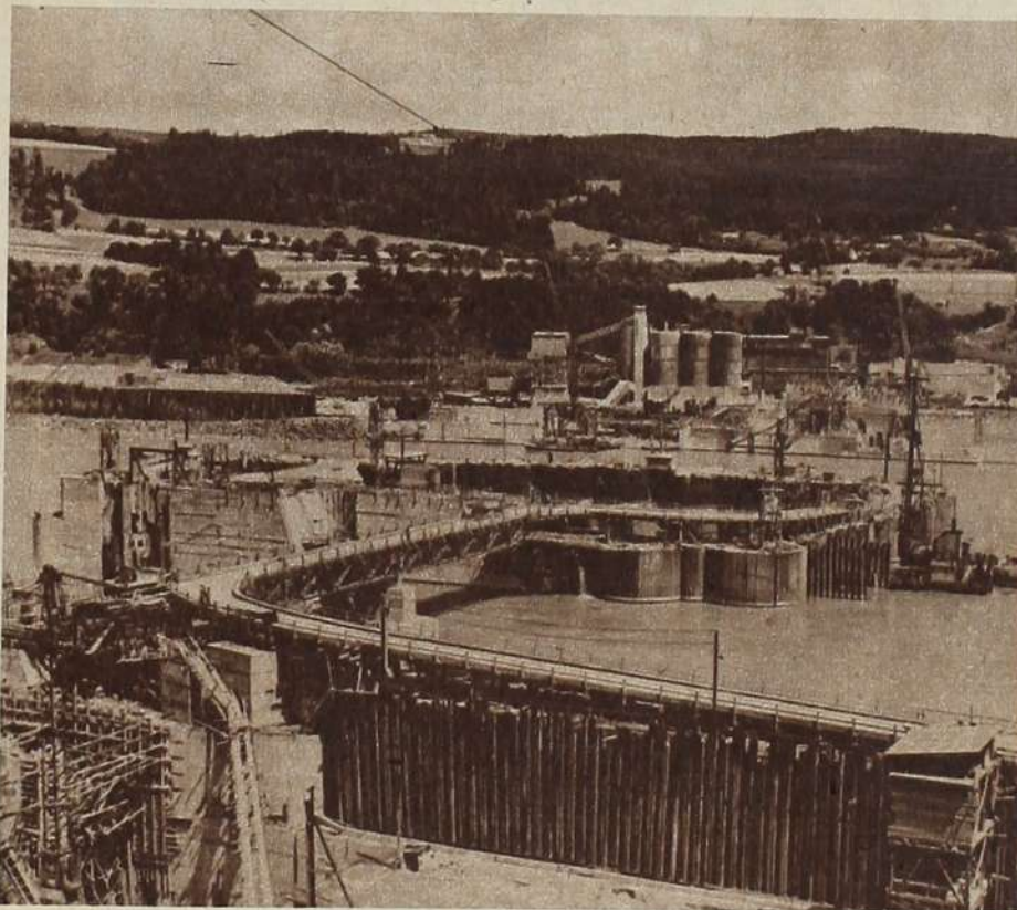
DER BAU DES DONAUKRAFTWERKS YBBS-PERSENBEUG macht große Fortschritte. Dieser Tage wurde eines der riesigen Schleusentore montiert. Schon Ende 1957 soll elektrischer Strom geliefert werden.
