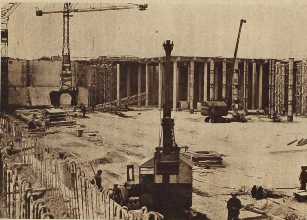
Die Kammern des Trinkwasserbehälters bei Neusiedl a. Steinfeld werden die bei derartigen Bauwerken noch nicht erreichte Fülltiefe von 10 m haben. Jede der 288 Säulen des Stahlbetonbauwerks trägt eine Last von 88 t.
