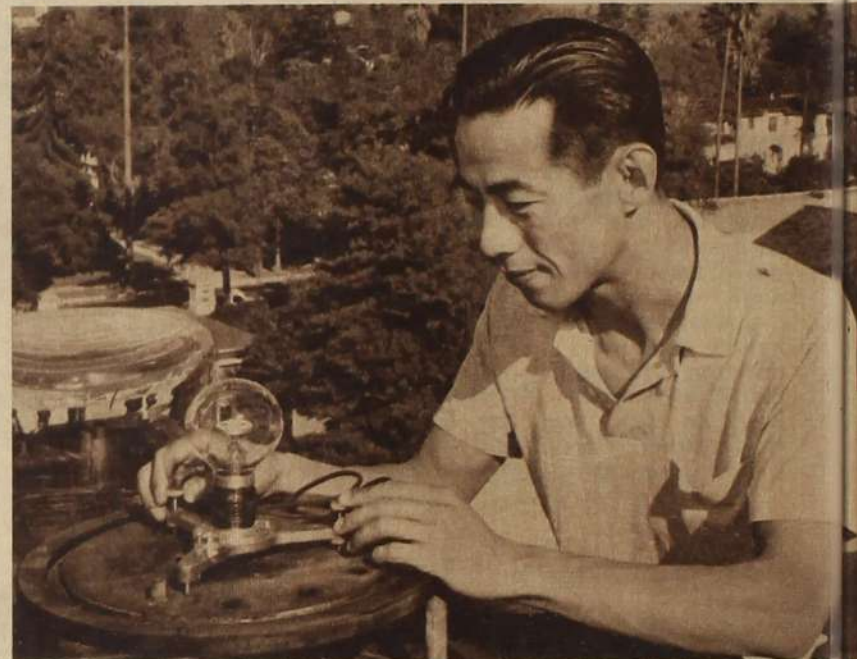
Dunst und Wolken beeinträchtigen die Leistungsfähigkeit des Sonnenofens. Vor Beginn der Arbeit bestimmt daher ein Wissenschaftler die zur Verfügung stehende Strahlungsenergie mit einem — Pyroheliometer genannten — Meßgerät.
