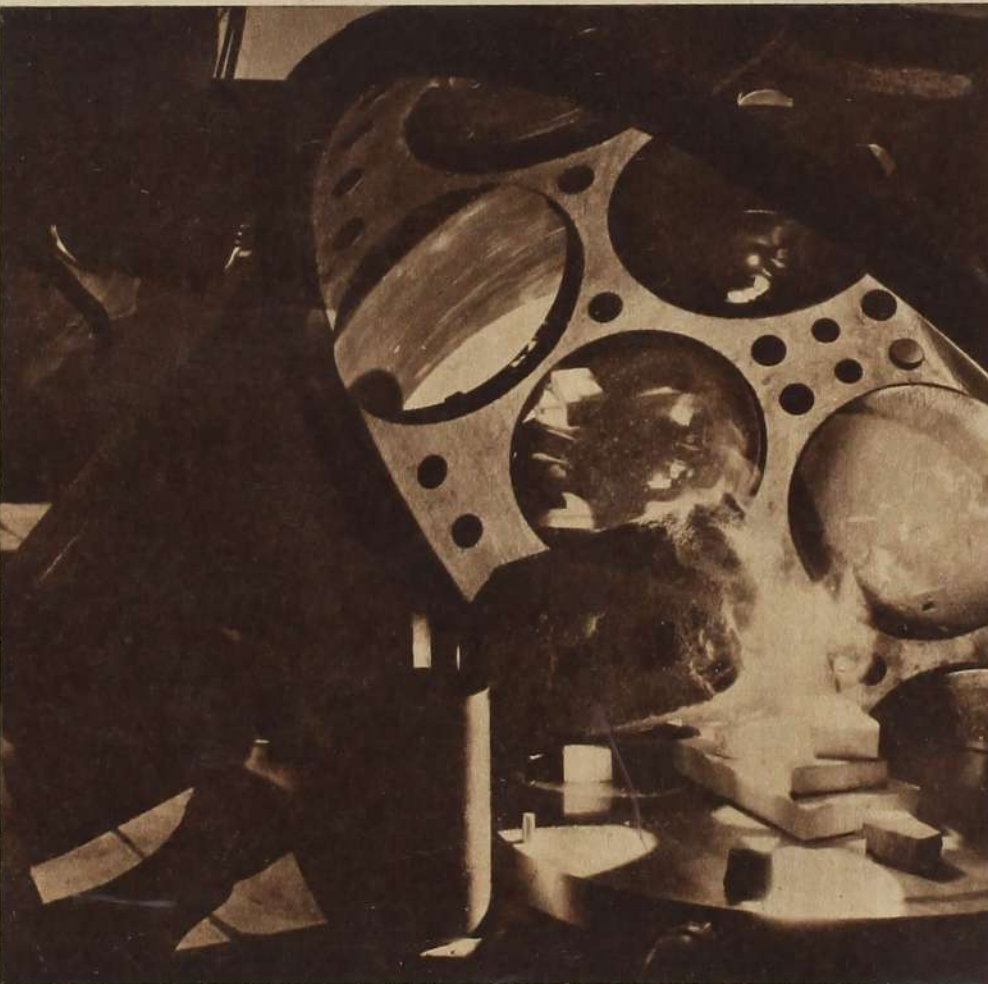
Wie ein riesiges Brennglas bündeln die 38 Linsen und 18 Spiegel des Sonnenofens die Sonnenstrahlen und erzeugen Temperaturen von mehr als 3000 Grad Celsius. Die Anlage, die in den Werkstätten der Technischen Hochschule von Kalifornien gebaut wurde, ist in ihrem fahrbaren Gehäuse auf der Kuppe eines Berges bei Pasadena untergebracht.
