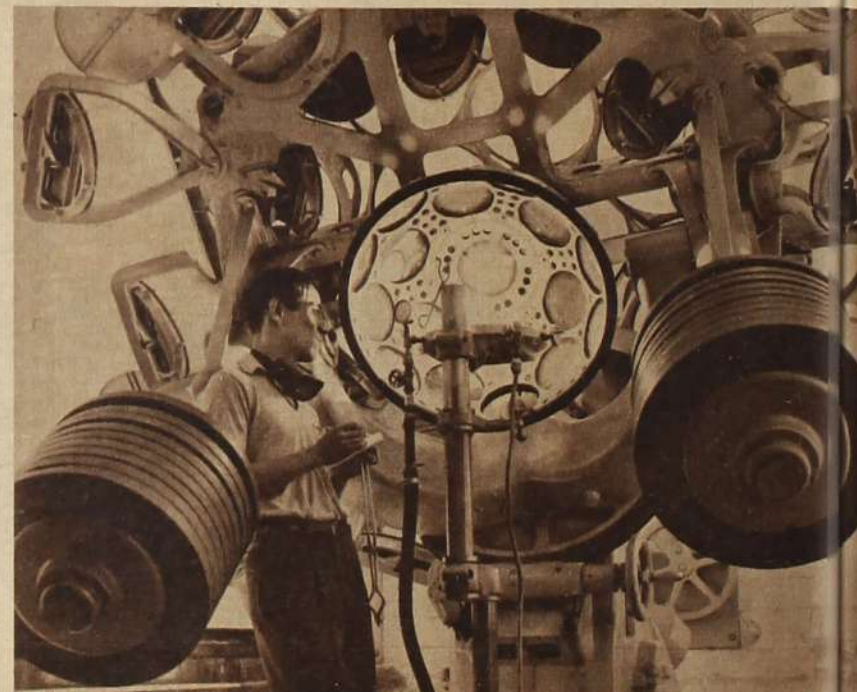
Dunst und Wolken beeinträchtigen die Leistungsfähigkeit des Sonnenofens. Vor Beginn der Arbeit bestimmt daher ein Wissenschaftler die zur Verfügung stehende Strahlungsenergie mit einem — Pyroheliometer genannten — Meßgerät.
