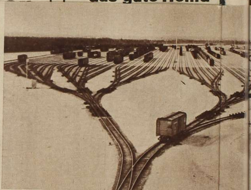
Der Rangierbahnhof Hamlet , Nordkarolina, besteht aus 120 Kilometern Gleisen. Die ankommenden Waggons werden automatisch auf eines der 58 Bestimmungsorte auf das gleiche Gleis kommen. Das Weichenstellen wird
