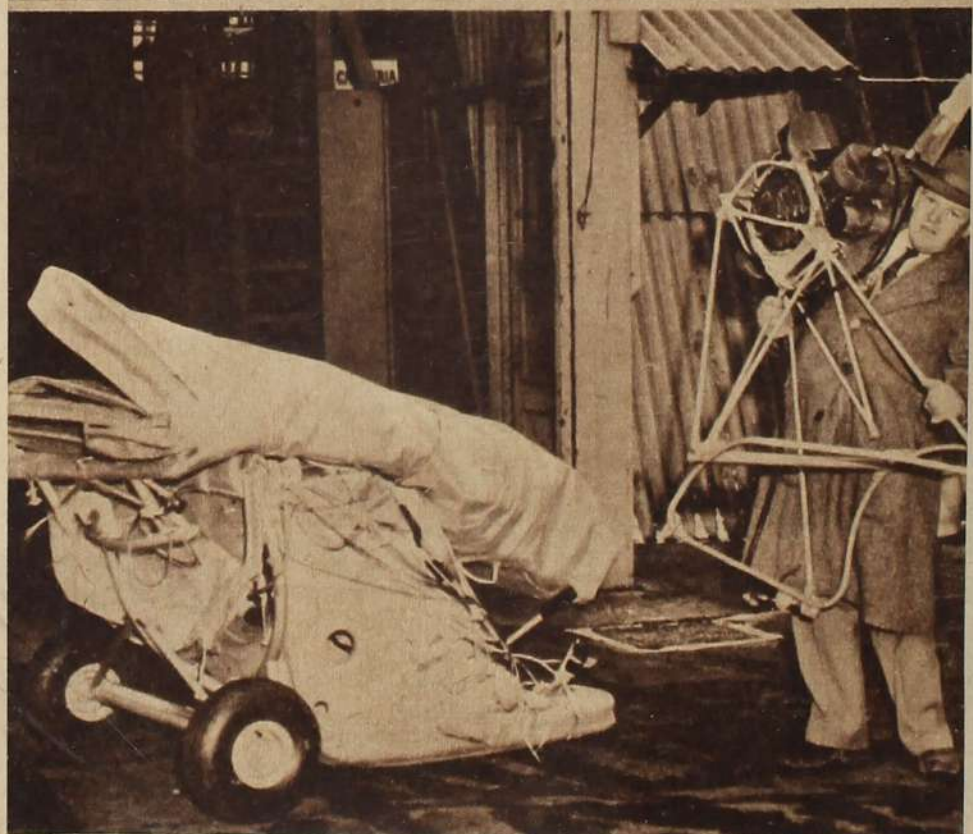
Im Kofferraum eines Personenwagens kann dieses Flugzeug untergebracht werden, das die Ingenieure der amerikanischen Firma Goodyear jetzt konstruiert haben. Tragflächen, Rumpf und Leitwerk — aus einem kautschuk-nylonartigen Stoff — lassen sich wie ein Ballon aufblasen, den Propeller betreibt ein 40 PS-Motor.
