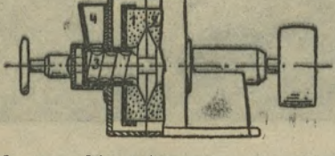
Abb. 2: Steinschrotmühle, teilweise im Schnitt. 1 = Fester Stein. 2 = Läuferstein. 3 = Schnecke zur Vorkonzentration. 4 = Einlauf.
